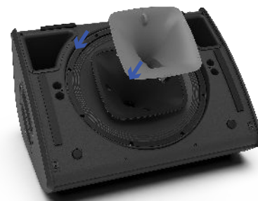
Une fois la grille retirée, des flanges magnétiques supplémentaires peuvent rapidement être installés de manière à changer la directivité pour passer de 60°x60° à asymétrique
