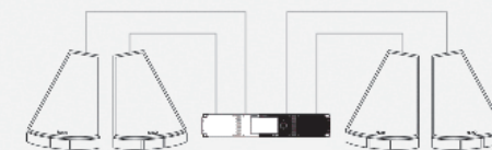
Système de retour de scène : 4 x 45°N12 amplifiés par NXAMP4X2MK2
